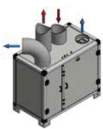
VERTICAL UVR-1/2 (con batería eléctrica PRE O POST)
