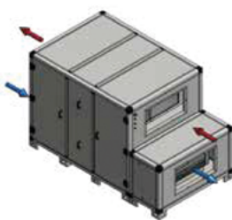
HORIZONTAL UVR-3/4/5/6 (con batería agua caliente/fría (70°/60°) (7°/12°)
