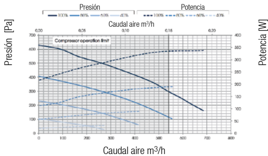
KRC HRU 3 EC / EX
