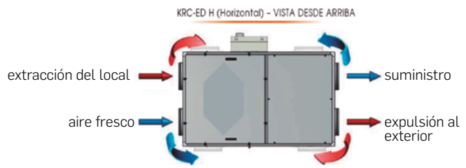
Configuración entradas - salidas
