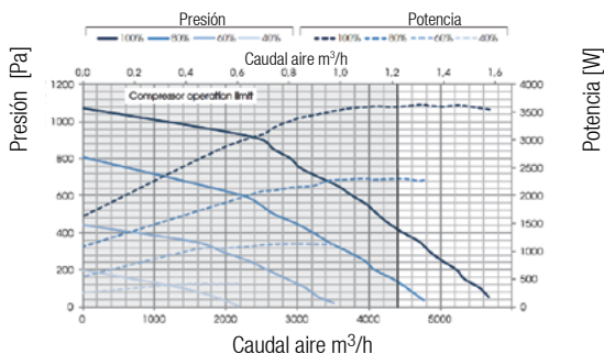
KRC HRU 5 EC / EX
