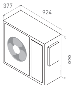
AQUARIS 04 / 06 / 08 kW
