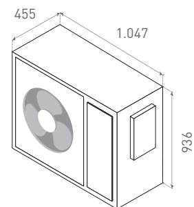
AQUARIS 10 / 12 kW
